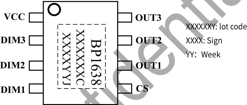
图 2 管脚封装图
